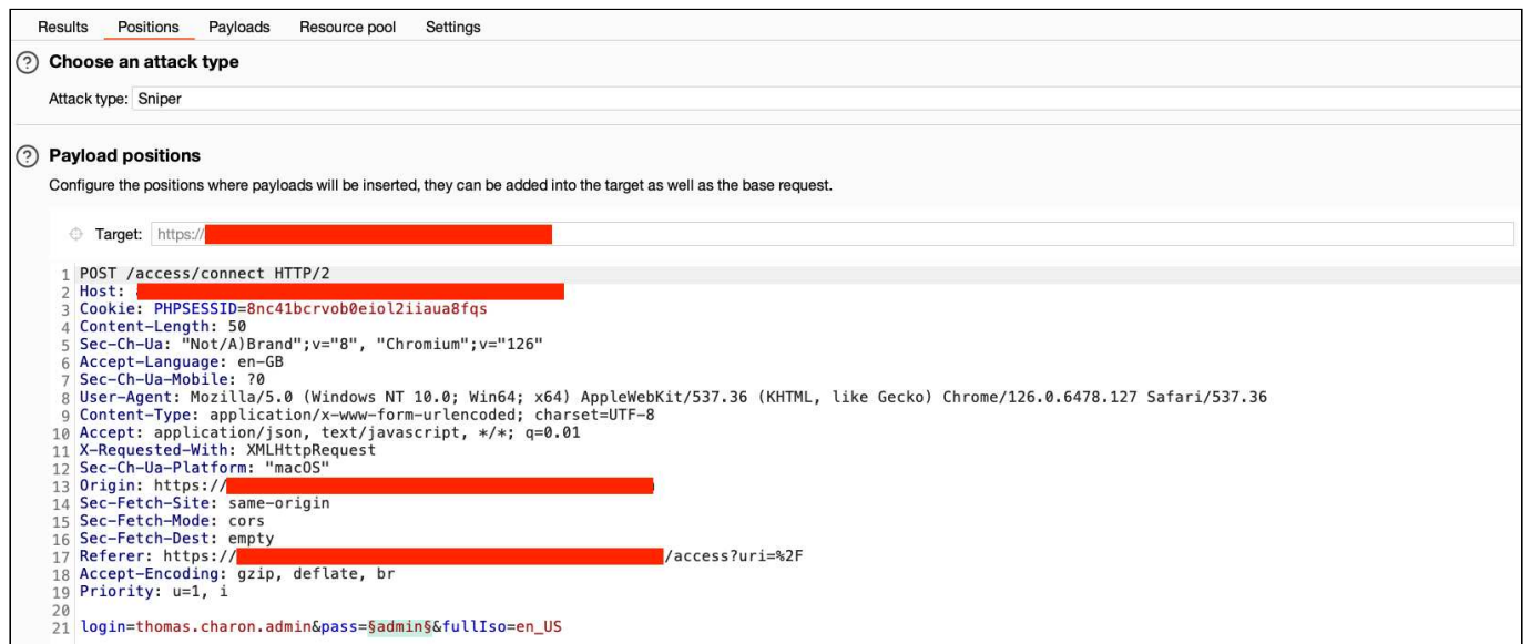
Figure 40 - Interface Burp Suite Intruder permettant de lancer une attaque par force brute sur le champ pass de la requête d'authentification
